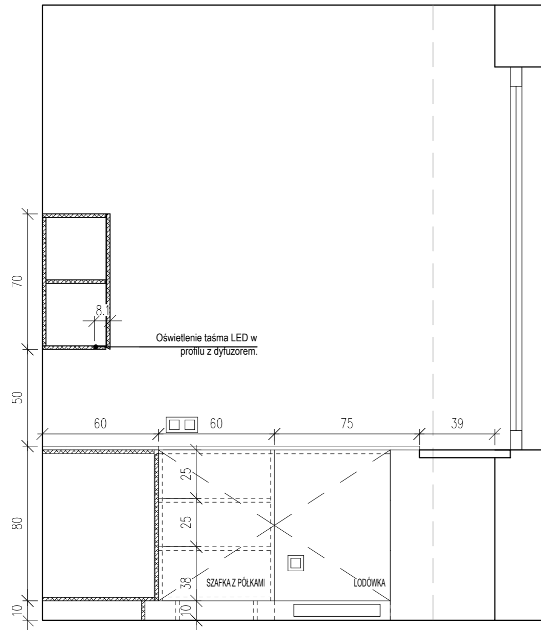
WIDOK B-B
