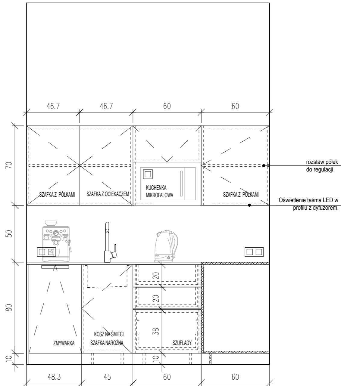
WIDOK A-A
