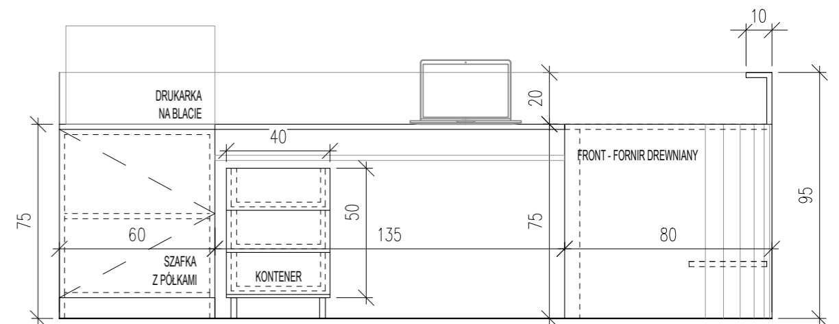
WIDOK D-D
