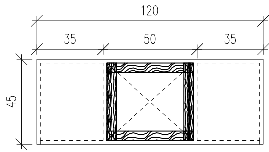
RZUT
