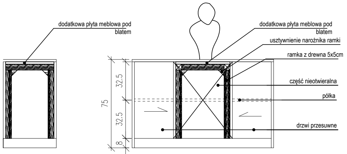
WIDOK
