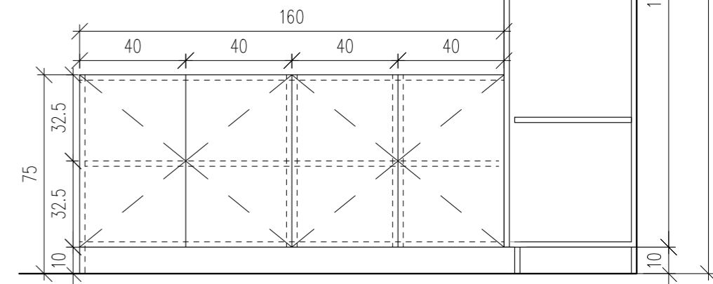
PRZEKRÓJ
