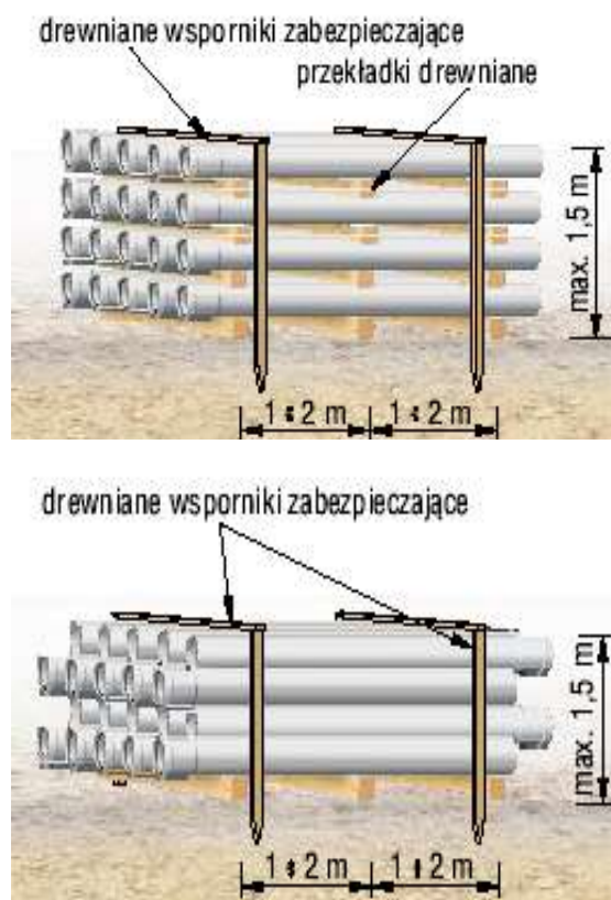
Rysunek poglądowy składowania rur PVC na placu budowy
